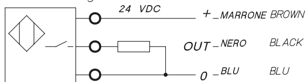
SCHEMA DI COLLEGAMENTO connection diagram
