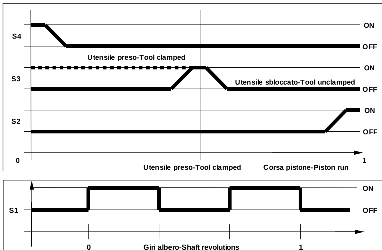
Diagramma di funzionamento sensori - Sensor working diagram
